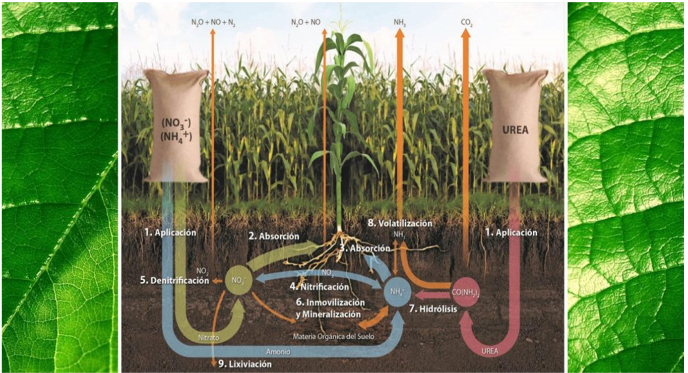
Figura nº 1: Ciclo del nitrógeno en el suelo.
